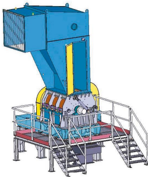
Le broyeur déchiqueteur à marteaux HM 100/100 PR
