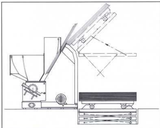
Equipement avec trémie pour alimentation par gravité, dispositif automatique empêchant un entassement de la matière ainsi qu'une ouverture d'entrée supplémentaire pour alimentation manuelle
