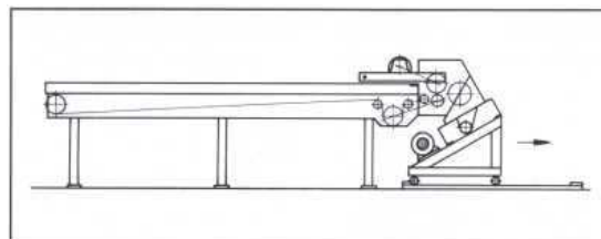
Broyeur avec dispositif d'avalement et bande convoyeuse pour alimentation horizontale de plaques
